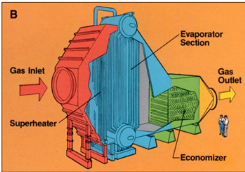
Drum over Drum Cross Flow HRSG
