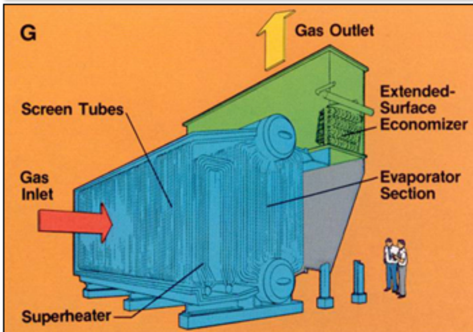
Drum over Drum Cross Flow w Screen Tubes HRSG
