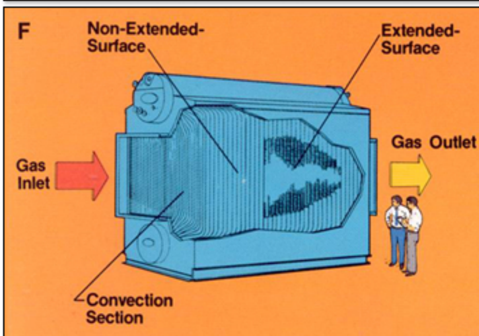
HRSG Factory Built Longitudinal Design
